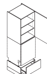
GGSa Geräteschränkbau für Geschirrspüler Appliance housing for dishwasher Armoire d'encastrement pour lave-vaisselle · Apparatenkastombouw voor vaatwasser → 60 ↓ 150/195/210/225
