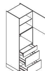
GBK Geräteschränk für Backofen Appliance housing for oven Armoire pour four Apparatenkast voor oven → 60 ↓ 150/195/210/225
