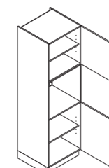
GB Geräteschränk für Backofen Appliance housing for oven Armoire pour four Apparatenkast voor oven → 60 ↓ 150/195/210/225
