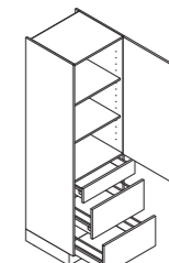
VAK Vorratsschränk Larder unit · Armoire à provisions Voorraadkast → 30/45/50/60 ↓ 150/195/210/225
