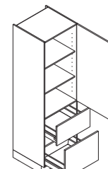
VZ Vorratsschränk Larder unit · Armoire à provisions Voorraadkast → 30/45/50/60 ↓ 150/195/210/225
