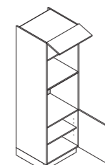
GBB Geräteschränk für Backofen und Mikrowelle Appliance housing for oven and microwave · Armoire pour four et micro-ondes · Apparatenkast voor oven en magnetron → 60 ↓ 150/195/210/225
